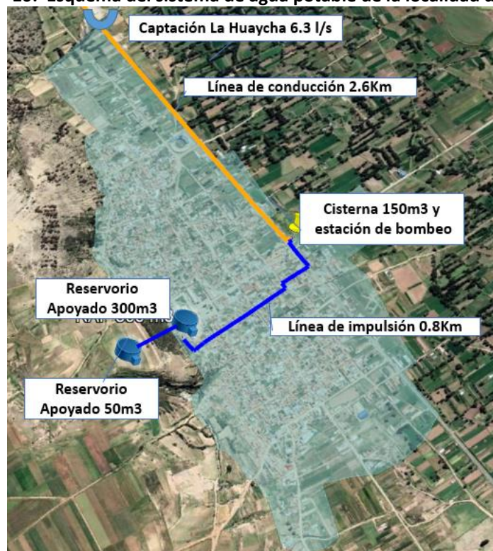
Imagen N° 10: Esquema del sistema de agua potable de la localidad de Orcotuna
