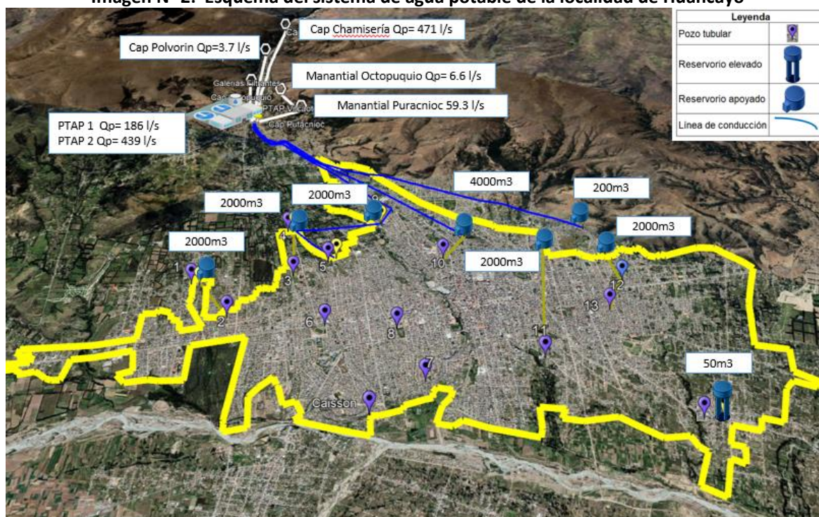
Imagen N° 2: Esquema del sistema de agua potable de la localidad de Huancayo
