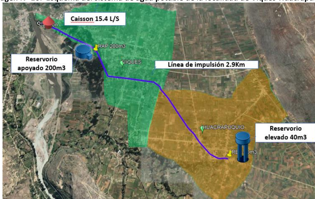
Imagen N° 16: Esquema del sistema de agua potable de la localidad de Viques-Huacrapuquio
